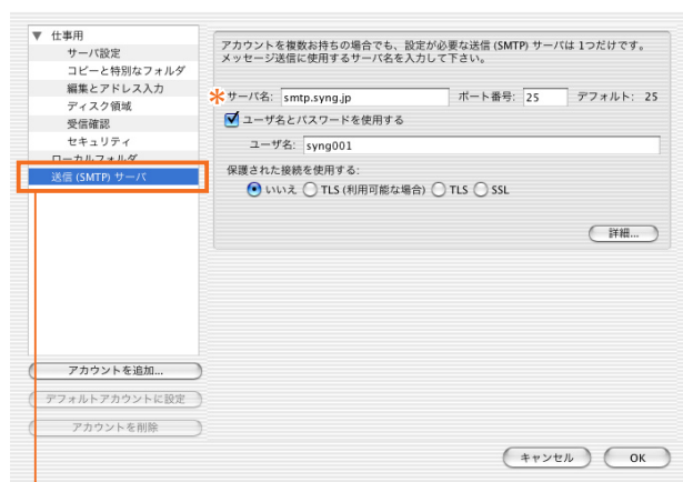
▼図：アカウント設定ダイアログ [送信 (SMTP) サーバ]メニュー
